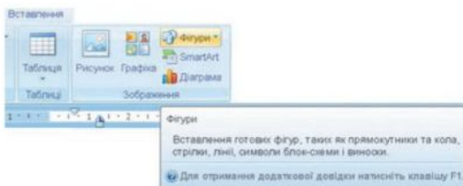
Рис. 4.35. Вставлення фігури
