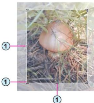
Рис. 3.42. Обтинання рисунка
