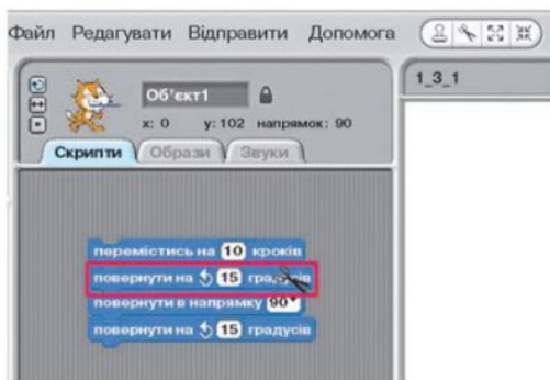
Рис. 1.22. Вилучення блока
