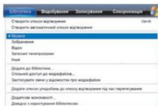
Рис. 3.27. Меню Бібліотека
